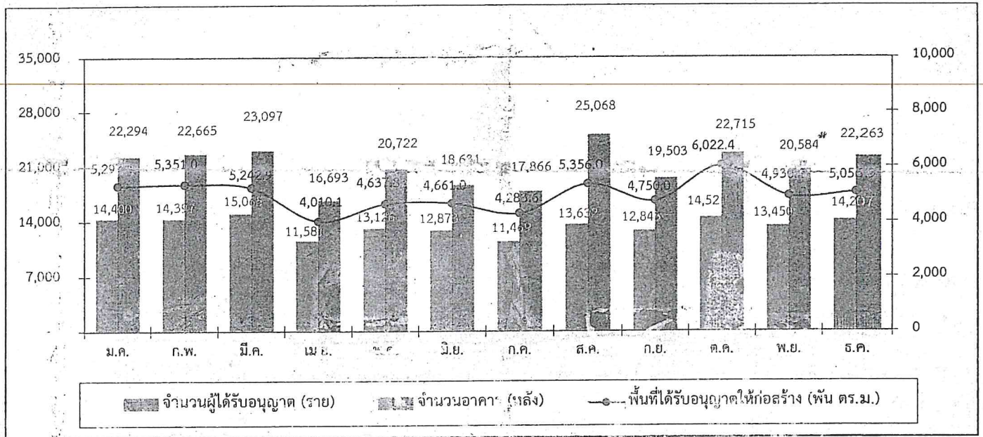
แผนภูมิ 1 จำนวนผู้ได้รับอนุญาตให้ก่อสร้าง จำนวนสิ่งก่อสร้าง และพื้นที่ก่อสร้างของอาคารโรงเรียน ที่ได้รับอนุญาตให้ก่อสร้าง ในเดือน มกราคม - ธันวาคม พ.ศ. 2562
